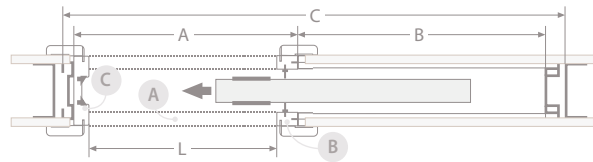
AZ EGYSZÁRNYÚ TOLÓAJTÓ MÉRTEI (mm)
