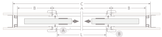
A KÉTSZÁRNYÚ TOLÓAJTÓ MÉRTEI (mm)
